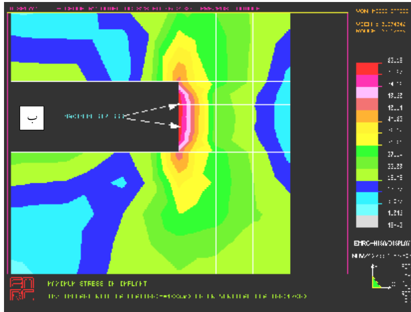
شکل ۵- تنش در ایمپلنت IMZ با پوشش هیدروکسی آپاتیت به ضخامت ۱۰۰ میکرون الف- توزیع تنش؛ ب- محل تنش ماکزیمم در ایمپلنت (قسمت فوقانی پیچ محکم‌کننده)
