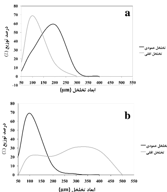
شکل (۲) - ابعاد تخلخل‌های عمودی و افقی در دو مقطع عرضی (a) طولی (b) داربست‌های PLGA/ژلاتین با استفاده از نرم‌افزار کمی تصویر
