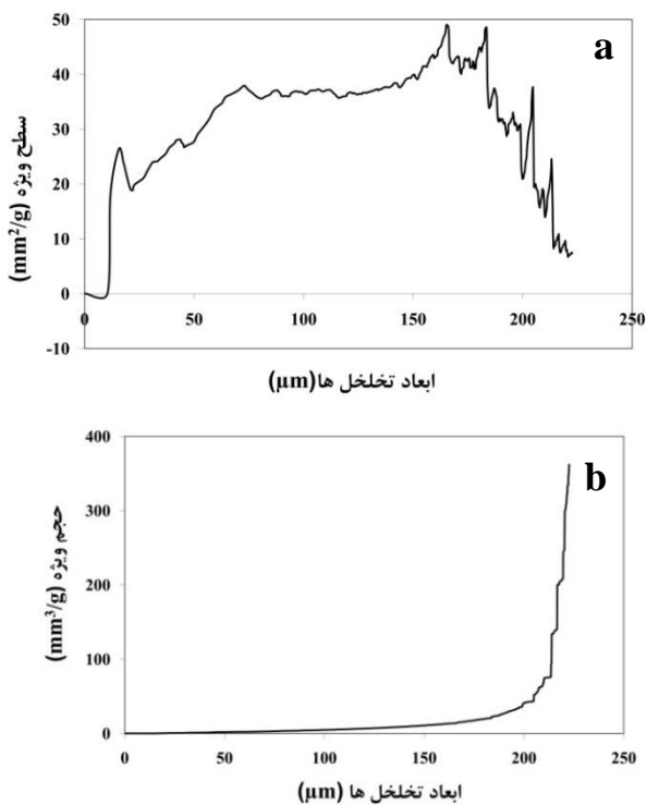
شکل (۳) - ابعاد تخلخل ها بر حسب سطح ویژه (a) و حجم ویژه (b) با استفاده از روش تخلخل سنجی جیوه‌ای
