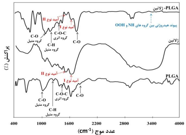
شکل ۴- طیف سنجی فرسرخ داربست‌های PLGA/ژلاتین ساخته شده به روش ریخته‌گری انجمادی
