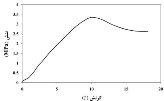
شکل ۵- استحکام فشاری داربست‌های PLGA/ژلاتین ساخته شده به روش ریخته‌گری انجمادی در جهت انجماد
