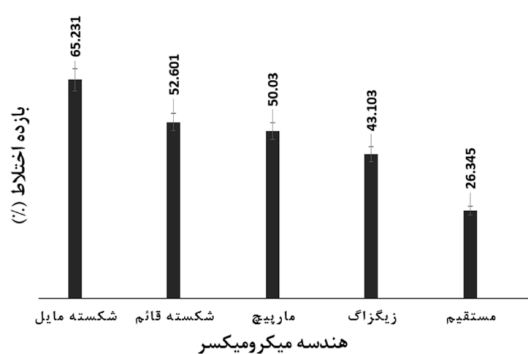
شکل (۵) - نمودار مقایسه‌ی بازده آزمایشگاهی میکرومیکسرهای
