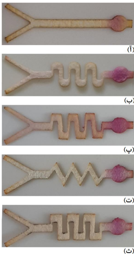
شکل (۴) - تشخیص نیتريت 10 \text{ mmolL}^{-1} در بزاق
