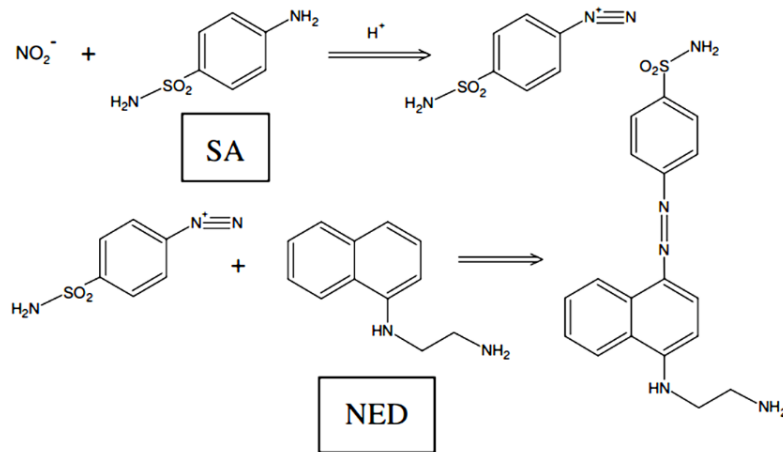
شکل (۳) - مراحل تشخیص نیتريت توسط واکنش گريس در يك محيط اسیدی [۲۲]
